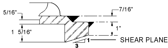
LONGITUDINAL SECTION "B-B"
